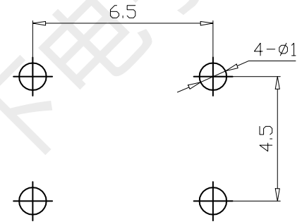
P.C.B焊接图
