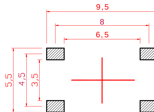
PCB. 焊接图
