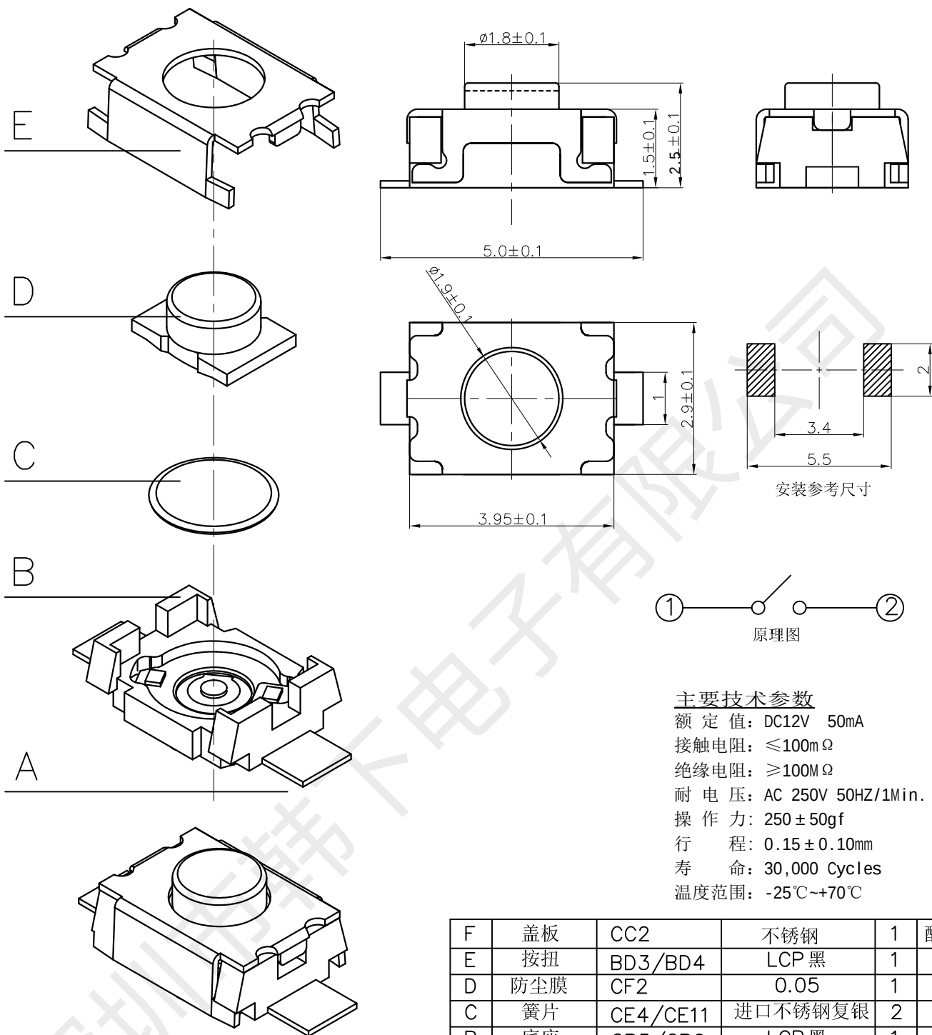
3D轴测图
