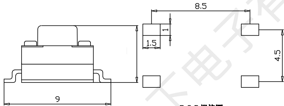
P.C.B焊接图
