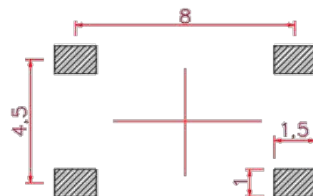
PCB. 焊接图
