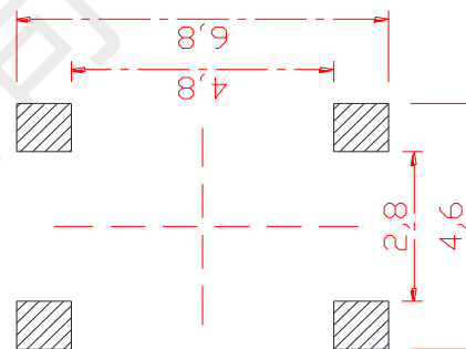
PCB. 焊接图
