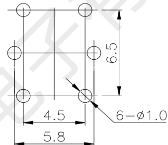
P.C.B LAYOUT
