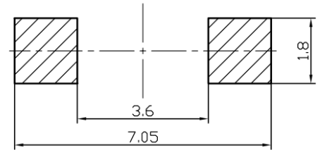
安装参考图
