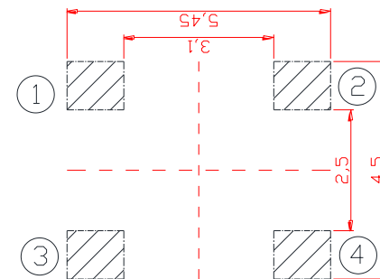
PCB. 焊接图
