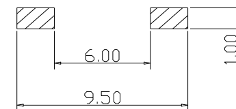
PCB. 焊接图
