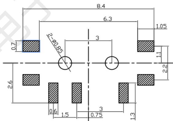
安装参考图
