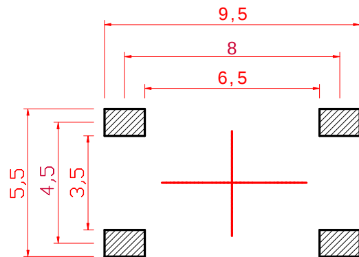
PCB. 焊接图
